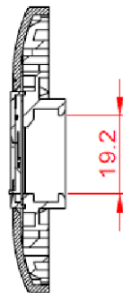
SECTION A-A
